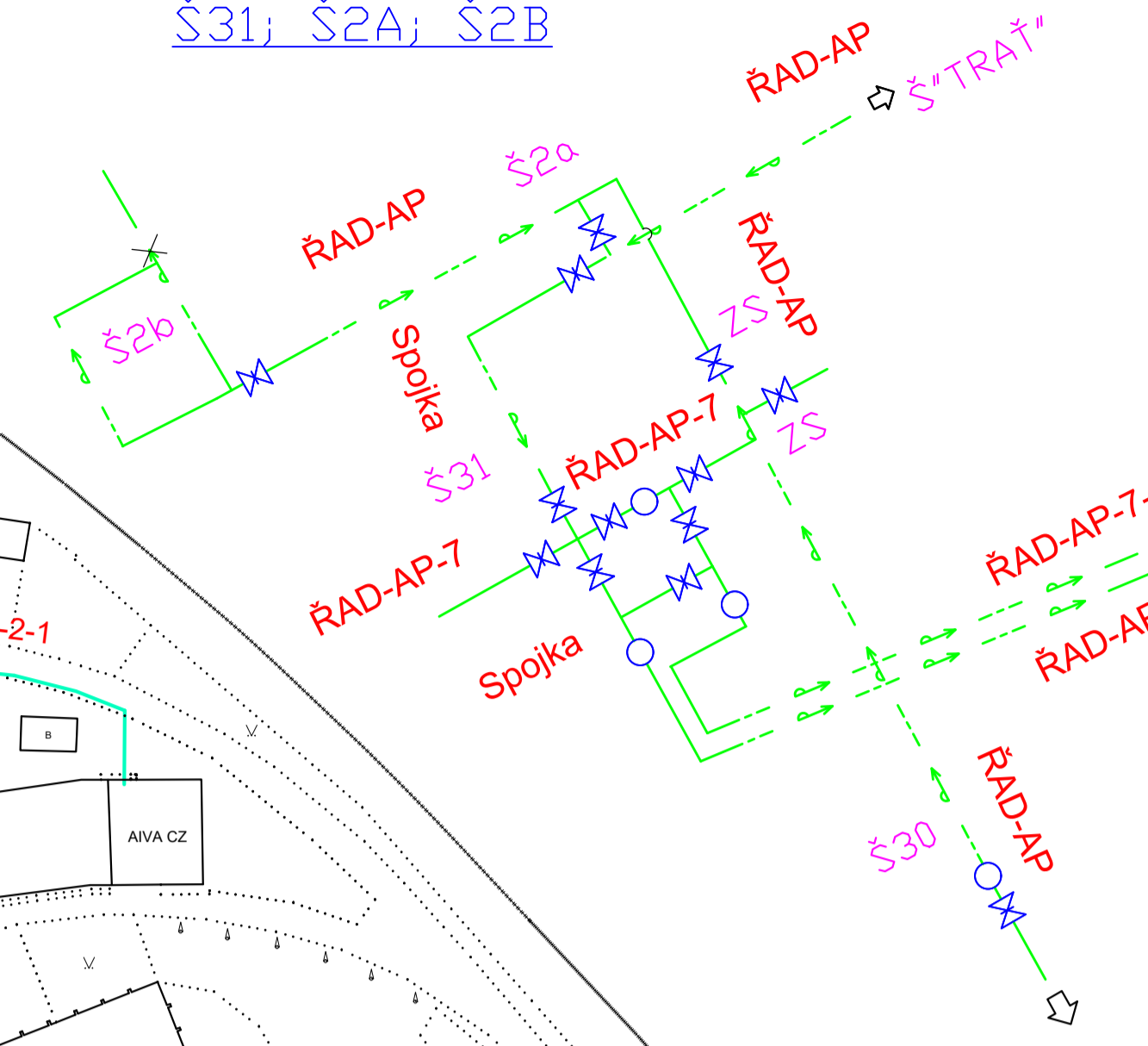
DETAIL ROZVEDU ŠACHTY Š31; Š2A; Š2B
