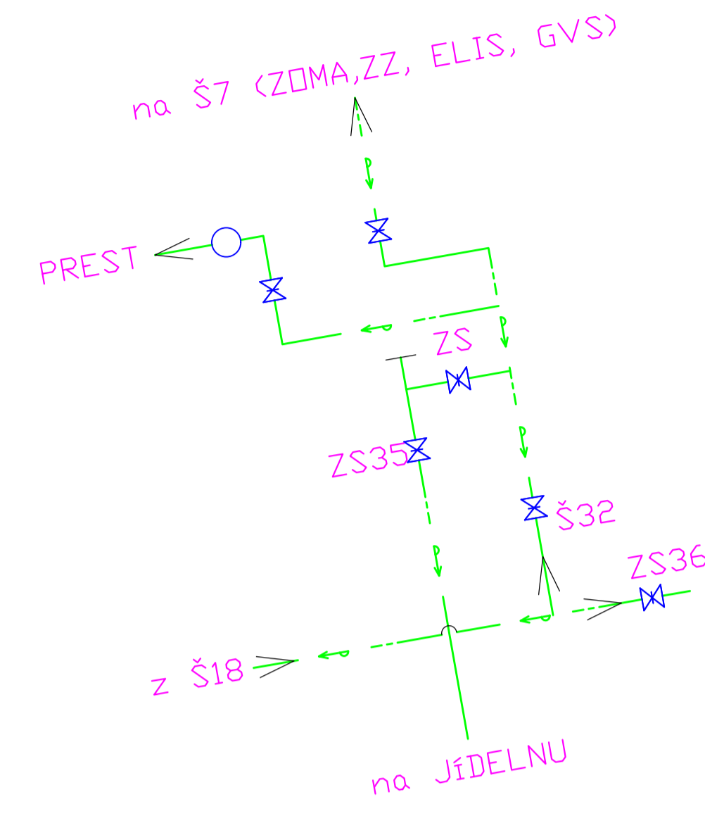
DETAIL ROZVEDU ŠACHTY Š32 a NÁPOJENÍ ŘADU AP3-3
