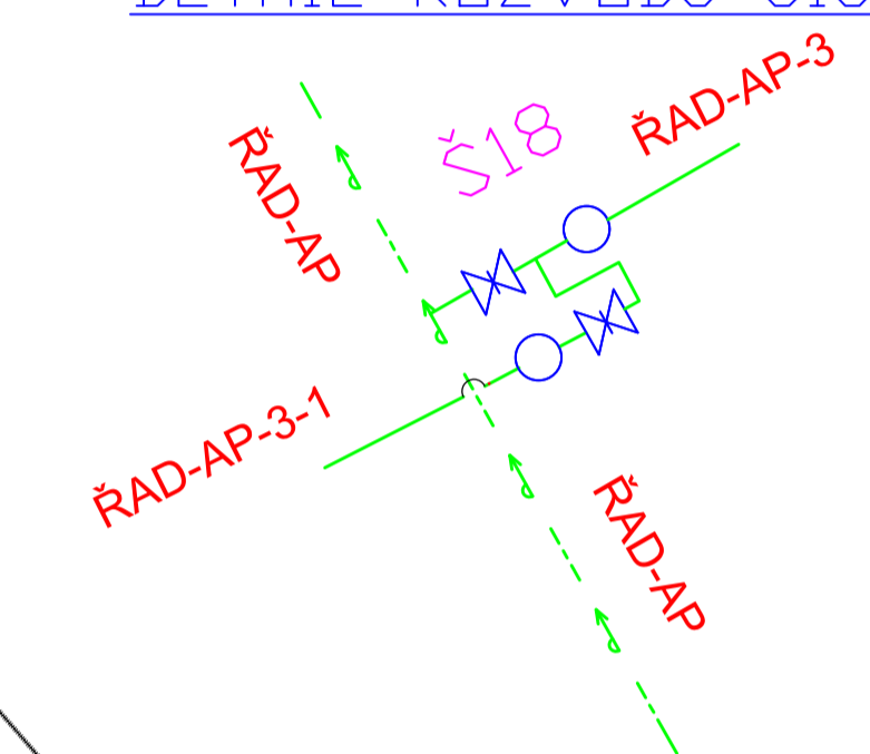
DETAIL ROZVEDU Š18
